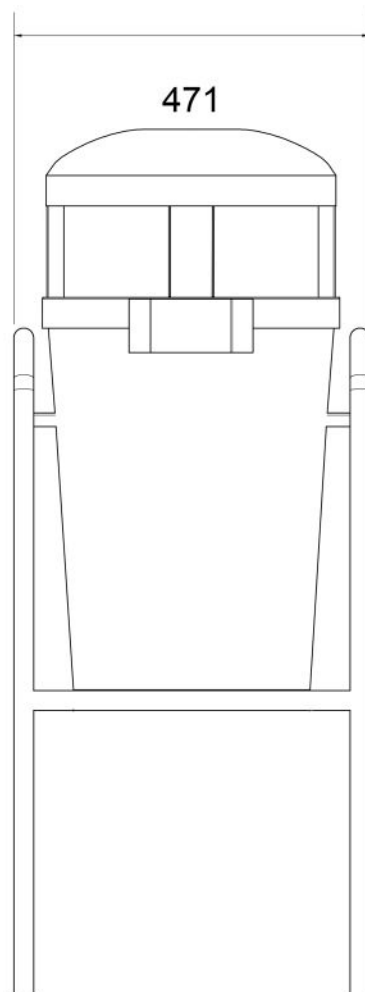
VISTA FRONTALE
