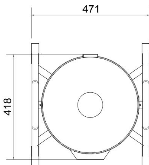
VISTA SUPERIORE
